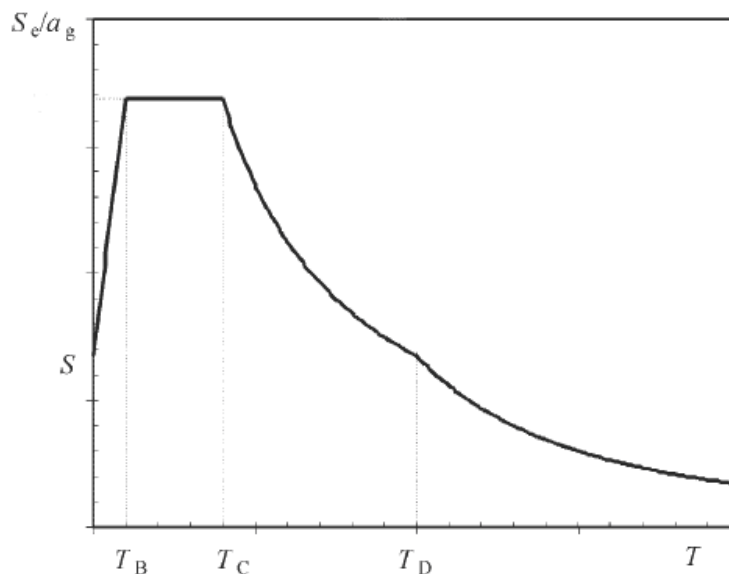
Dimensieloos elastisch responspectrum uit NPR (fig 3.1)
